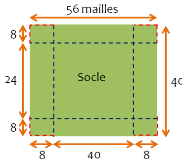
Plan d'un socle Longueur : 56 mailles Largeur : 40 mailles
