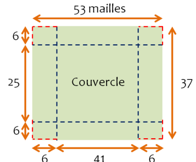
Plan d'un couvercle Longueur : 53 mailles Largeur : 37 mailles
